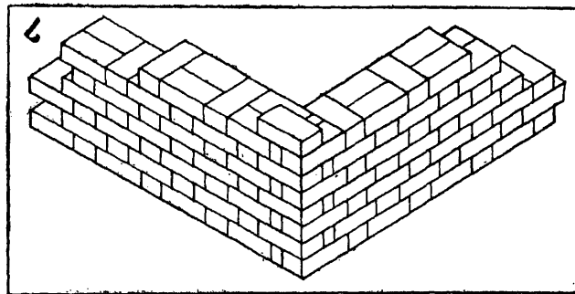
८. Flemish bond : फ्लेमिश. ९. Flemish garden bond or Sussex : फ्लेमिश गार्डन किंवा ससेक्स.
